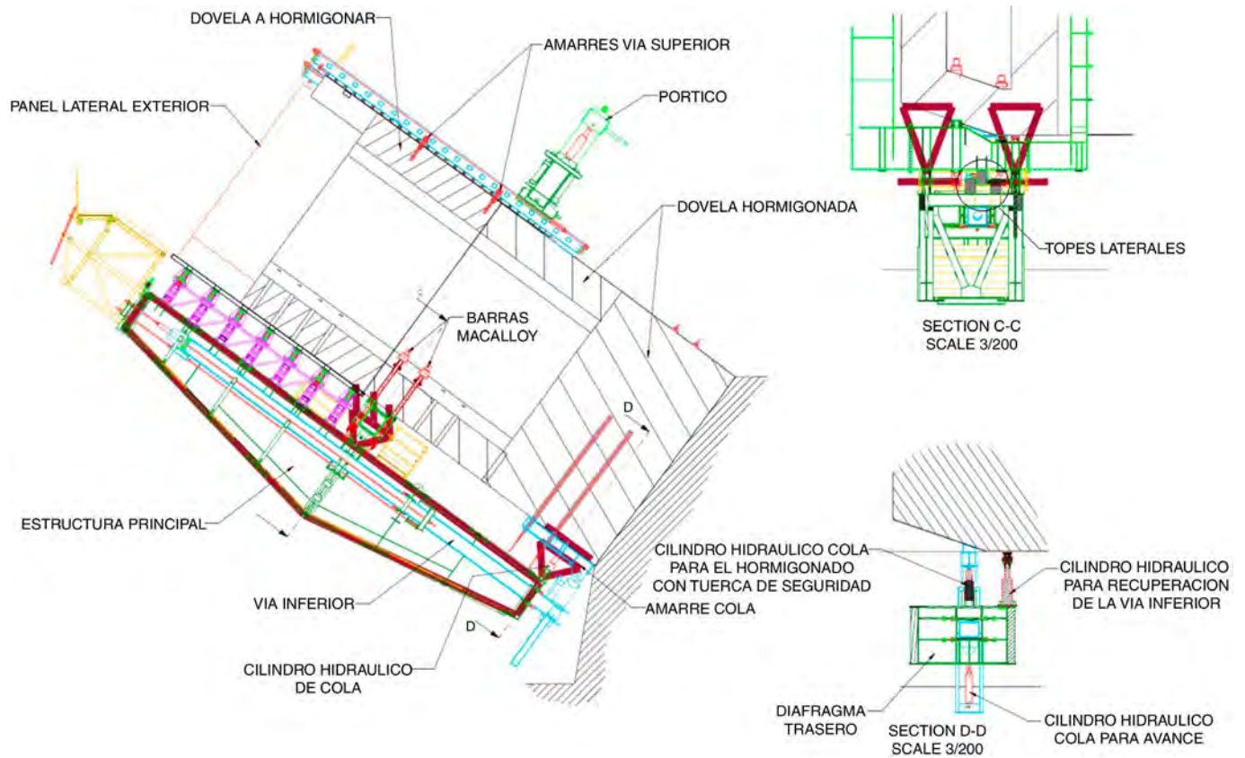
Figura 7. Esquema estático: fase de de hormigonado.
