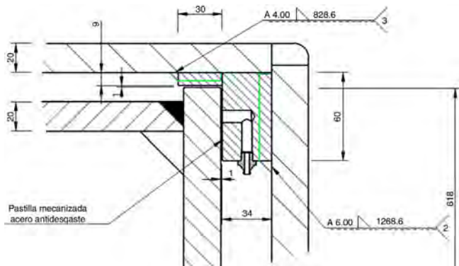
Figura 6. Detalle de contacto en pieza deslizante
